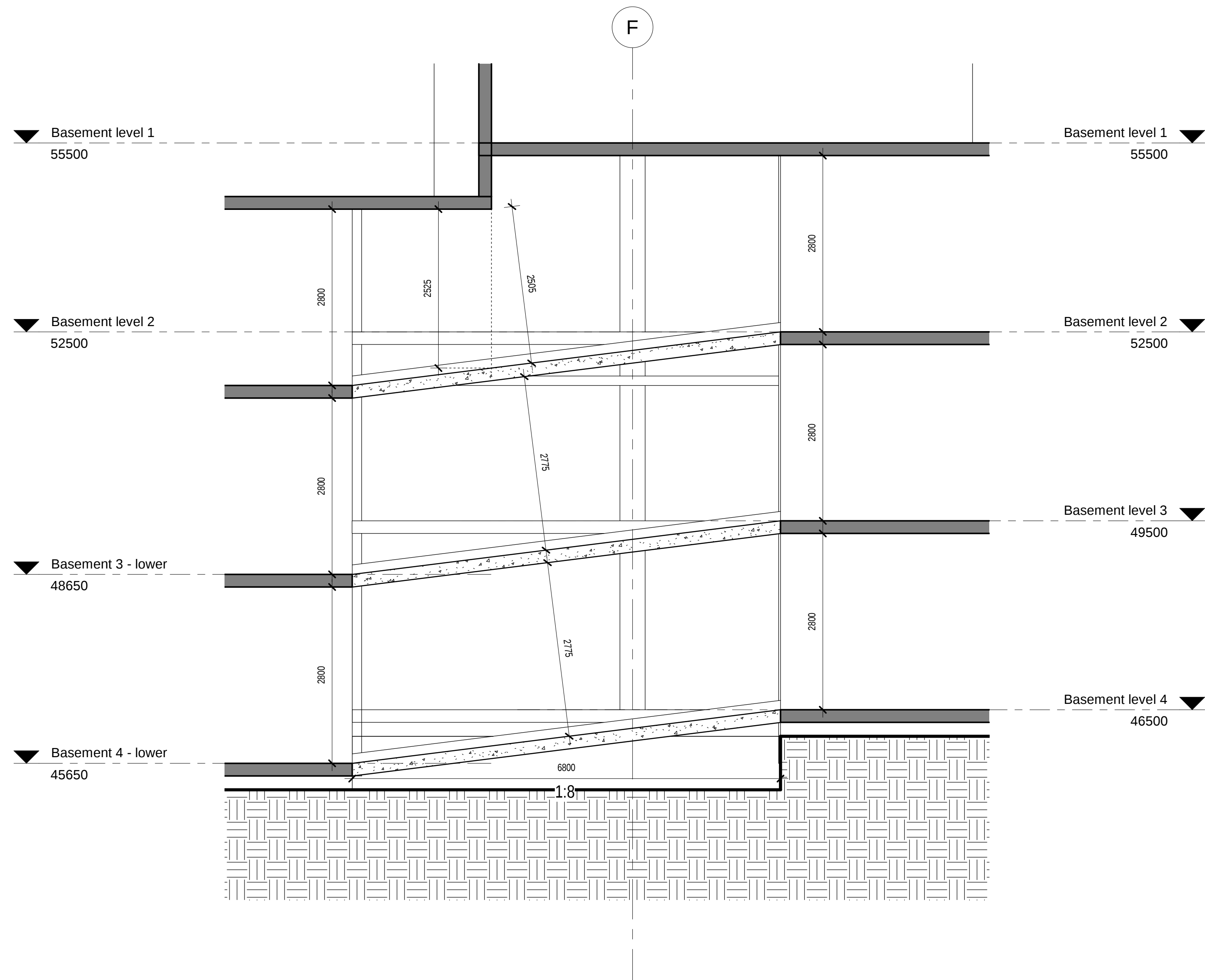
1 Ramp 2 1 : 50
