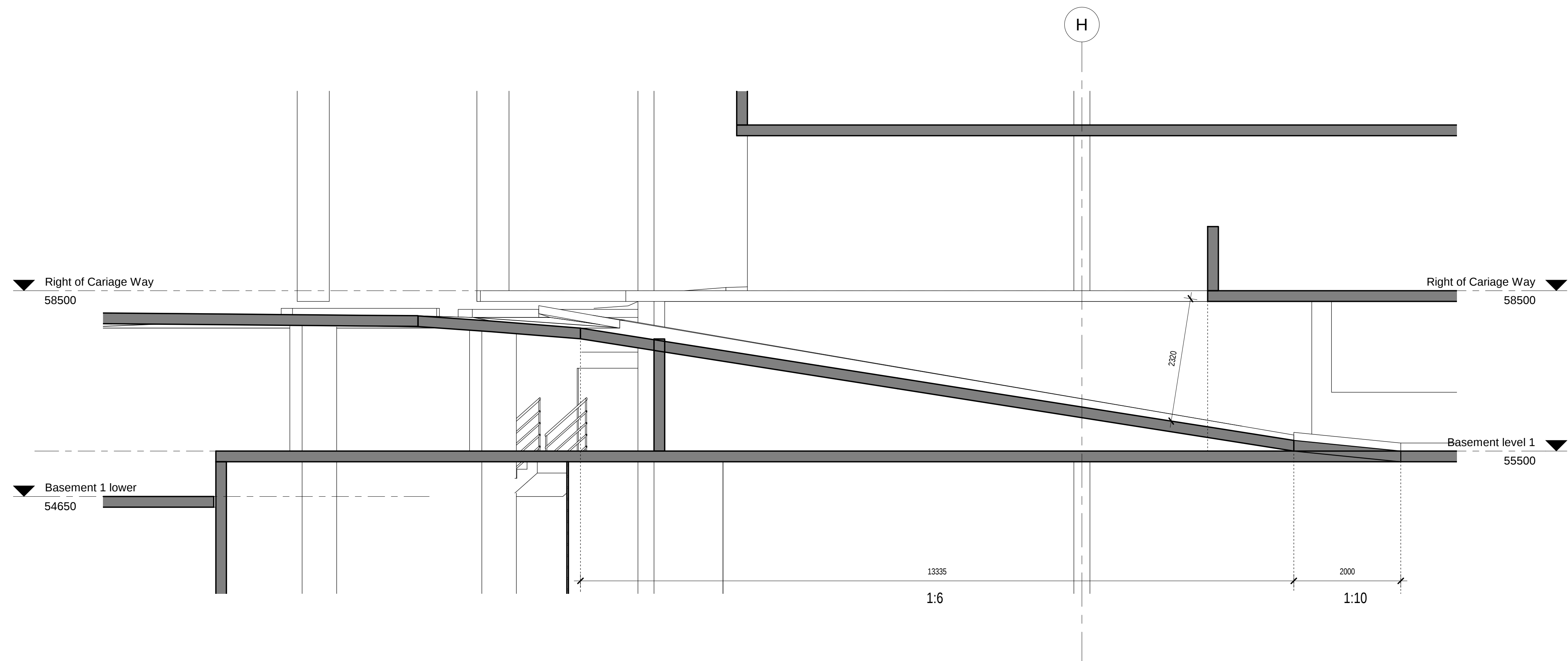
1 Ramp 3 1 : 50
