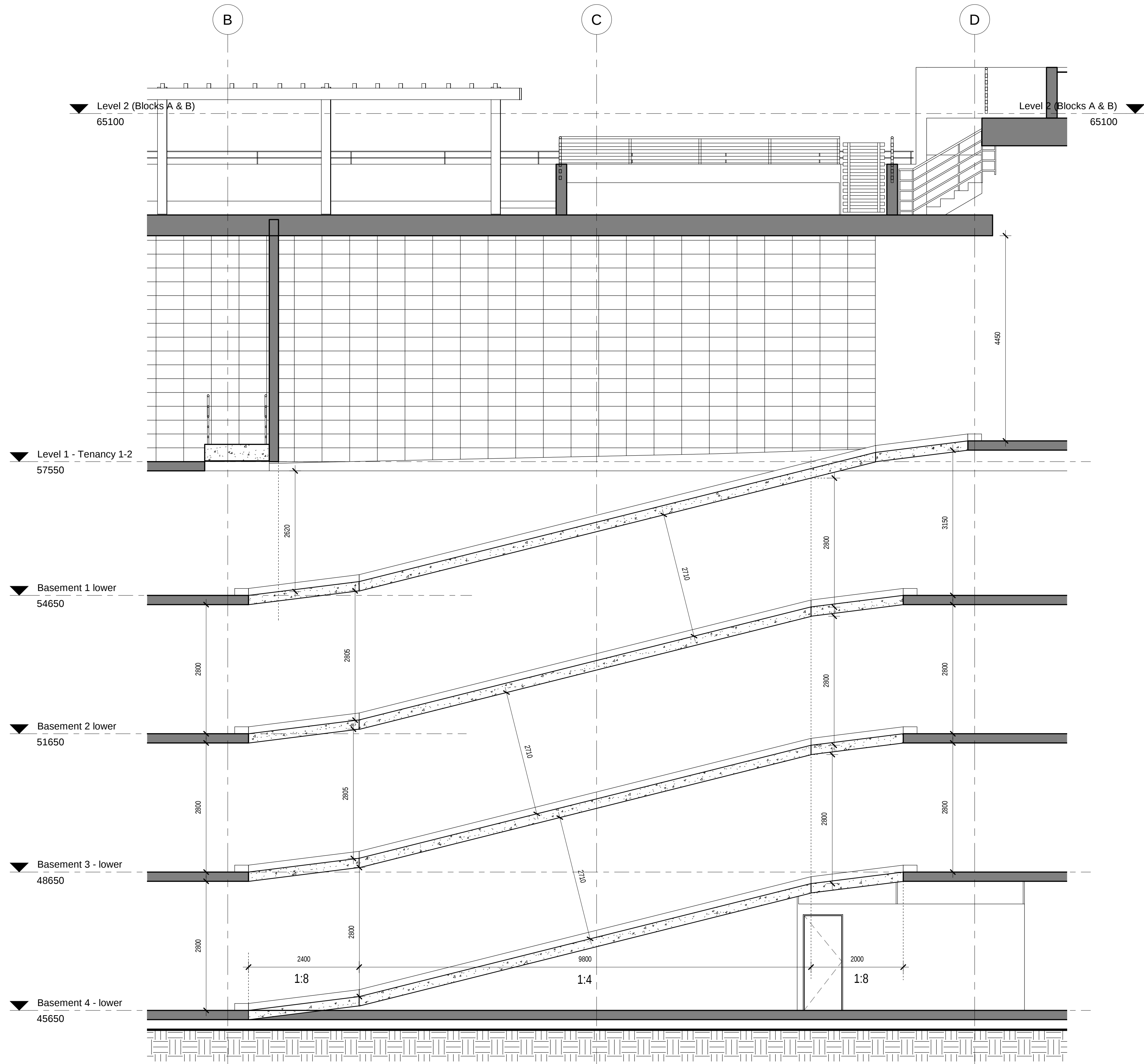
1 Ramp 1 1 : 50
